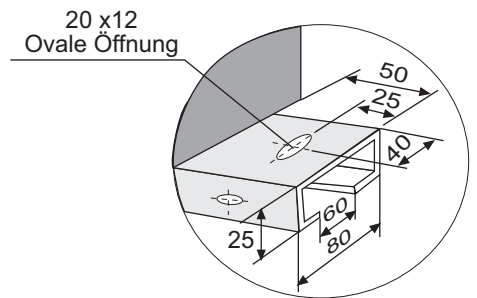
Detailzeichnung Halterung f. Geräteverankerung
