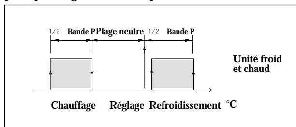
Fig. J – Fonctionnement unité froid + chaud.
