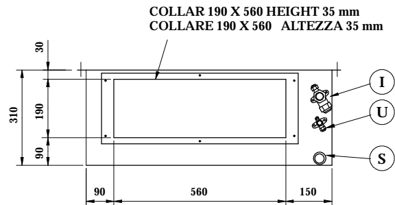
REAR VIEW / VISTA POSTERIORE Rectangular duct version / Versione con collare rettangolare
