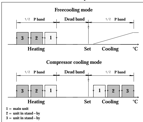
Fig. L – Sistema composto da 3 unità totali, di cui 2 in stand-by – Controllo Microface
