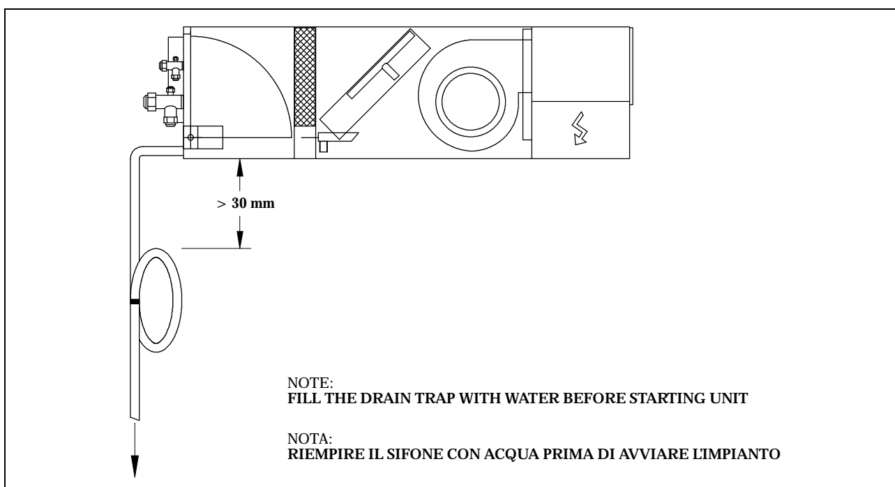
Fig. 10 – Condensate drain / Scarico condensa
