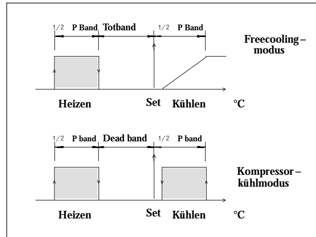
Abb. K – Betrieb des Kompressors, der Heizregister und der Öffnung der Freecooling-Regelklappe
