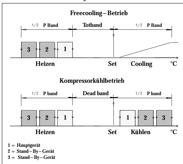
Abb. L – System aus 3 Gesamtgeräten, 2 davon im Stand-By – Microface – Regler
