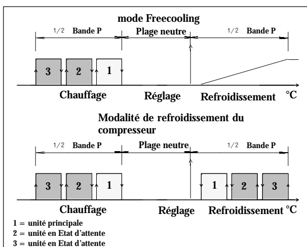
Fig. L – Système constitué de 3 unités totales, dont 2 en Etat d'attente – Unité de commande Microface
