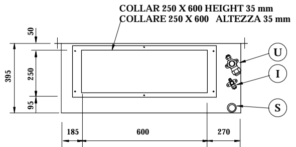
REAR VIEW / VISTA POSTERIORE Rectangular duct version / Versione con collare rettangolare
