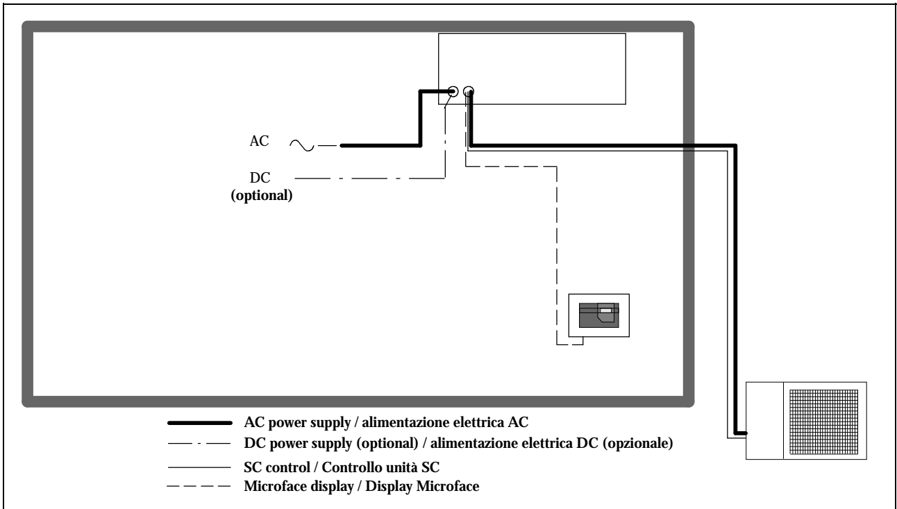
Fig. 6 – Electrical connections / Collegamenti elettrici
