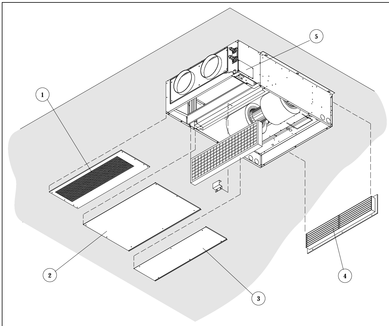
Fig. 12 – Maintenance example / Esempio di manutenzione
