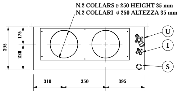
REAR VIEW / VISTA POSTERIORE Circular ducts version / Versione con collari circolari
