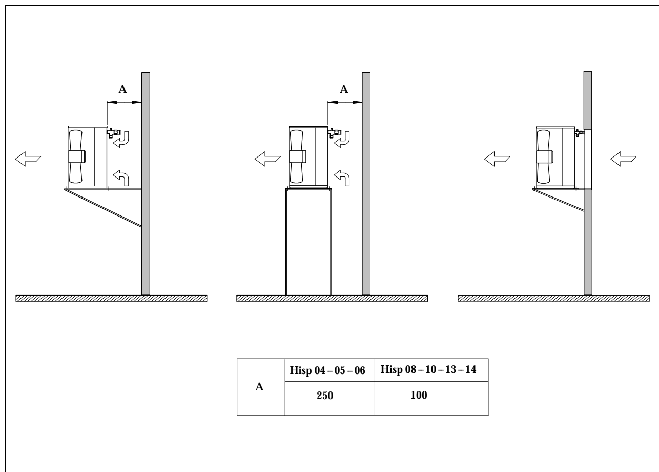
Fig. 3 – Condenser positioning / Posizionamento unità condensante
