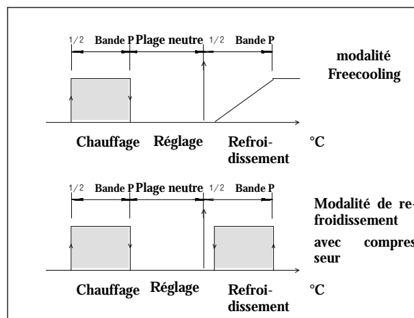
Fig. K – Fonctionnement du compresseur, résistances électriques et ouverture du rideau de Freecooling
