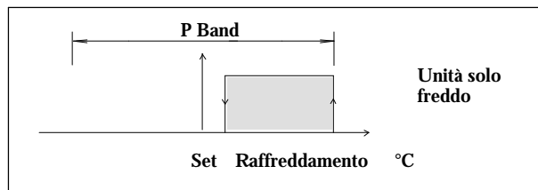
Fig. 1 – Funzionamento unità solo freddo.
