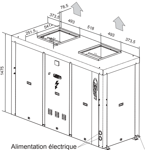
PARTIE CONDENSATION
