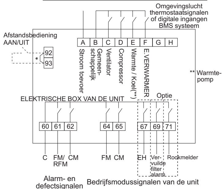
DUBBELE CIRCUIT UNIT, VFC VERSIE
