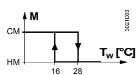
Automatische Umschaltung
