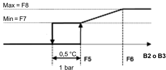
Abb. 3 : Kondensationsgebläse-Regelung
