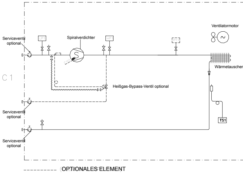
LAUßENEINHEITRIOR KSC M 22E/26E/32E/38E/43E
