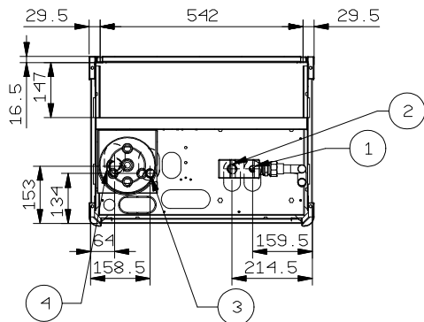
SEZ. A - A
