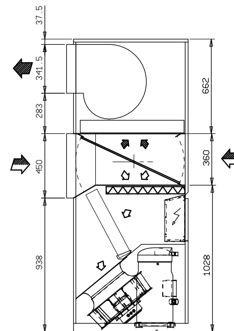
SEZ. A-A STANDARD VERSION
