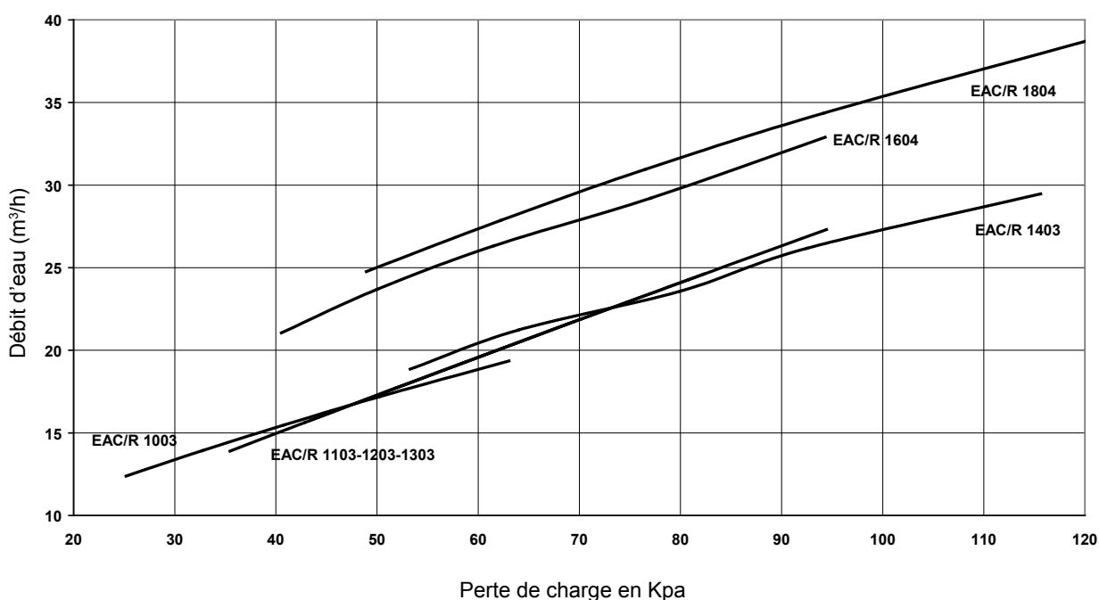
PERTE DE CHARGE + FILTRE À EAU (*)
