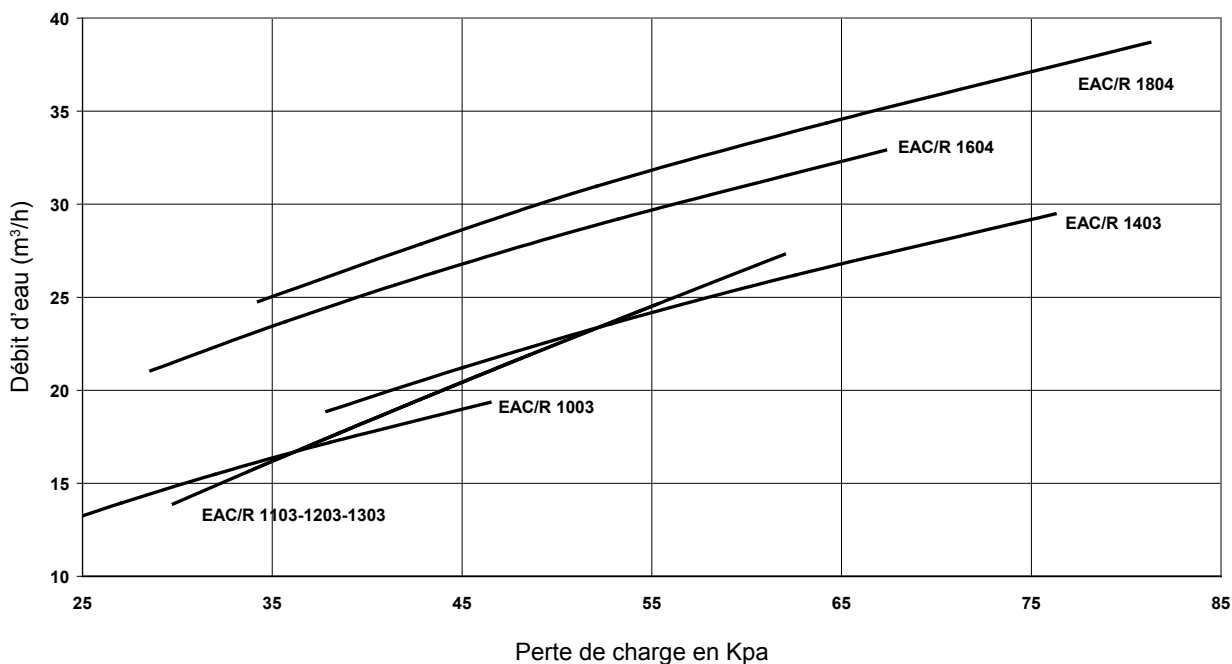
PERTE DE CHARGE SANS FILTRE
